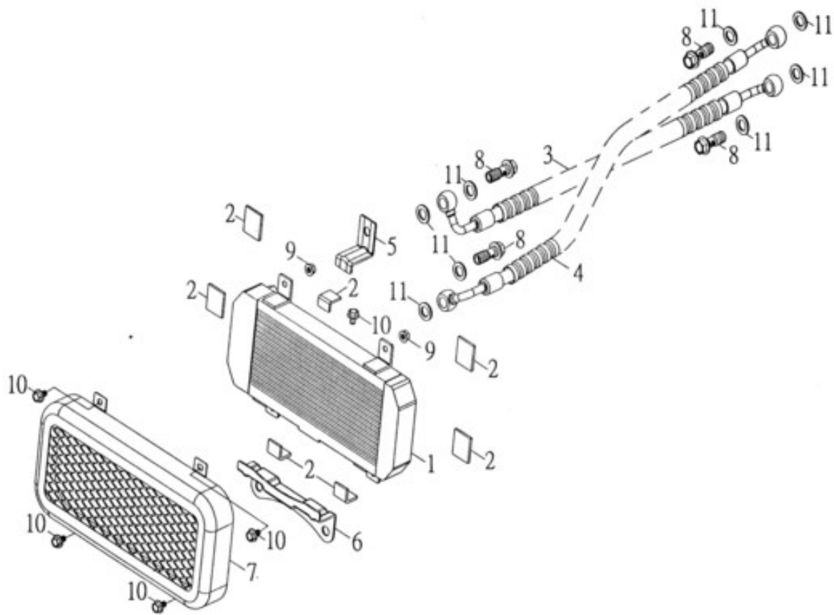
FIG.38 RADIATOR 油冷卻器
